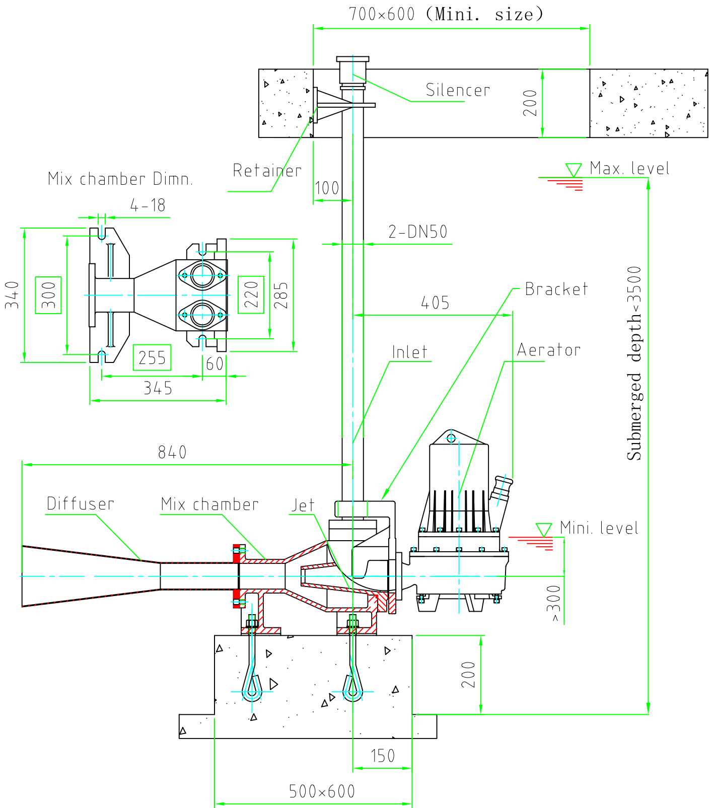
QSP3 Dimn.
