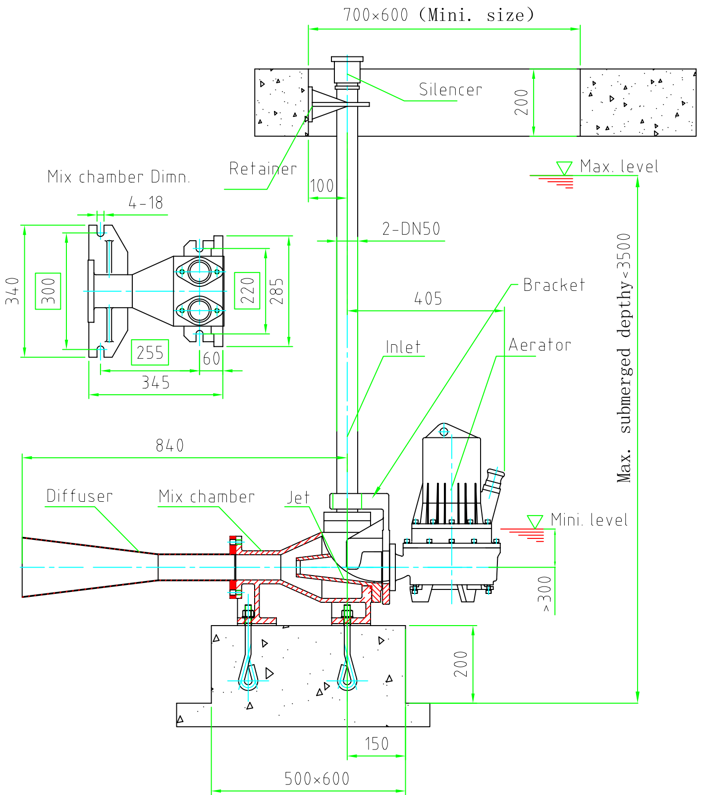
QSP2.2 Dimn.
