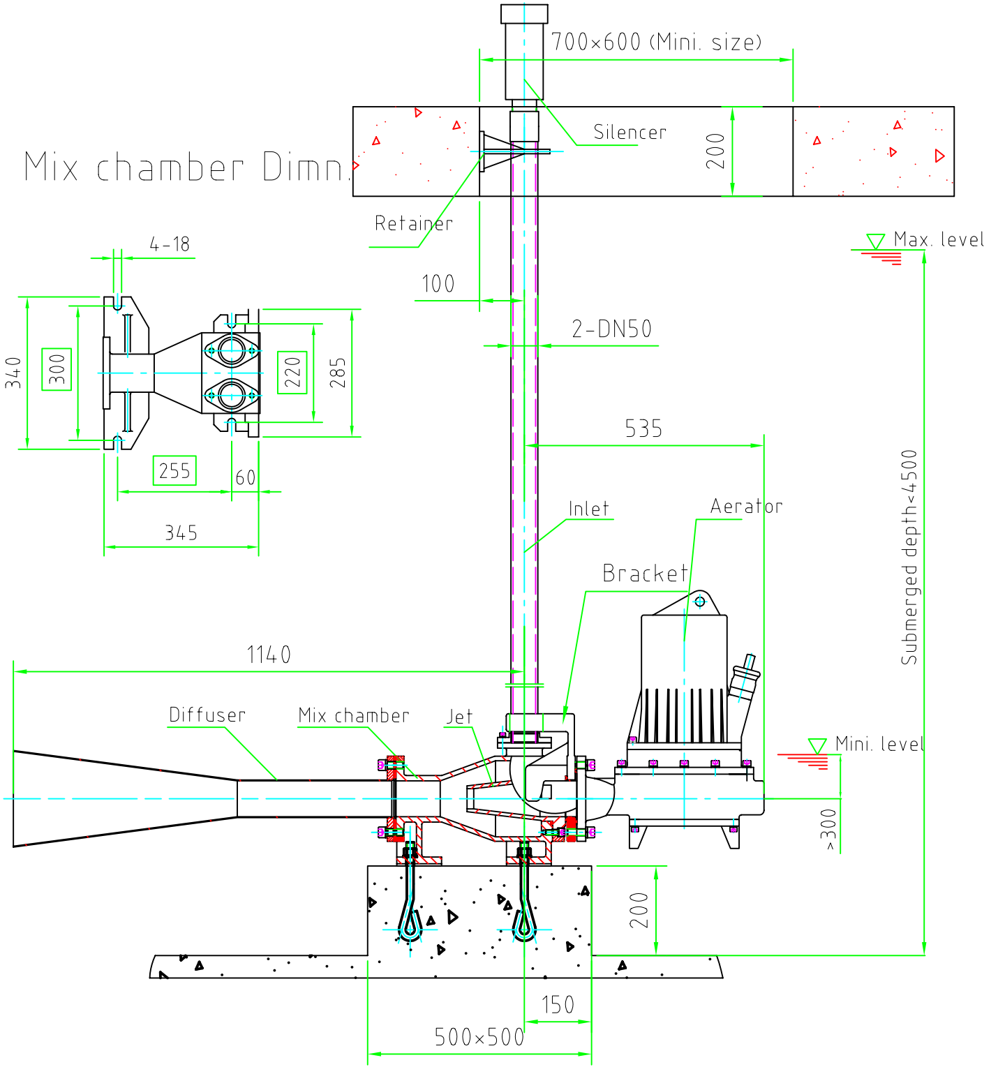
QSP4 Dimn.
