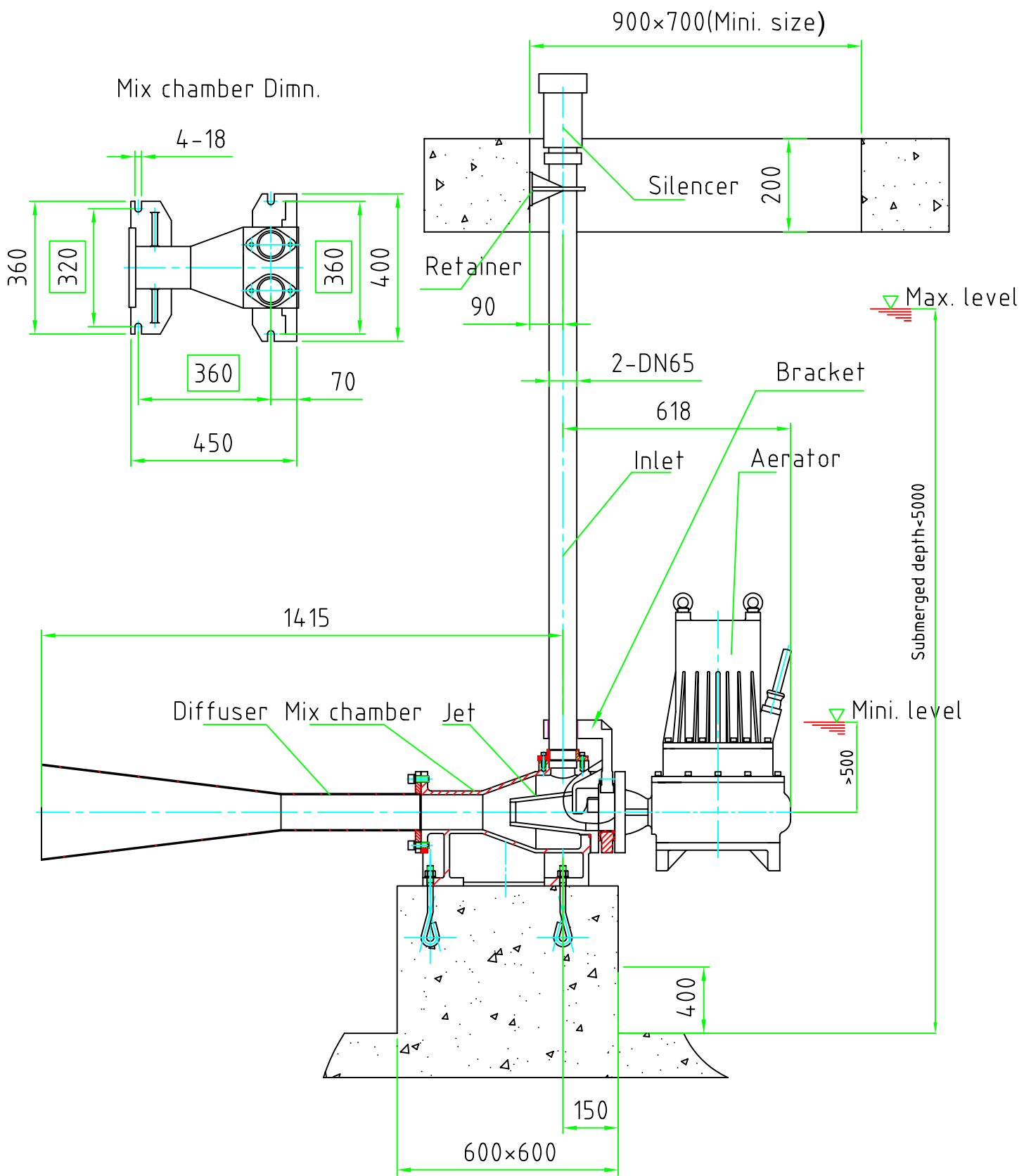
QSP5.5 Dimn.
